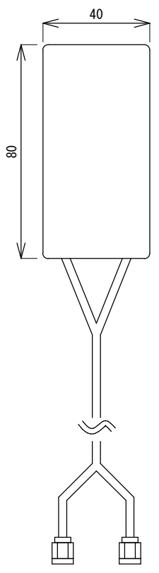
LTEアンテナ L=5.5m
