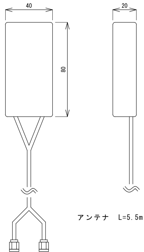
メール通信制御装置 DM-2
