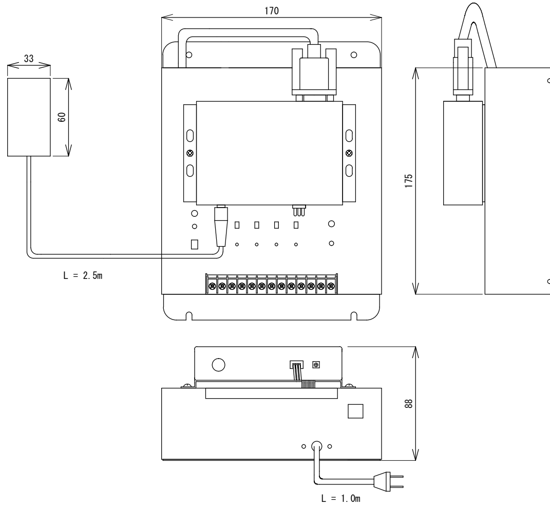
メール通報装置 KEm-103
